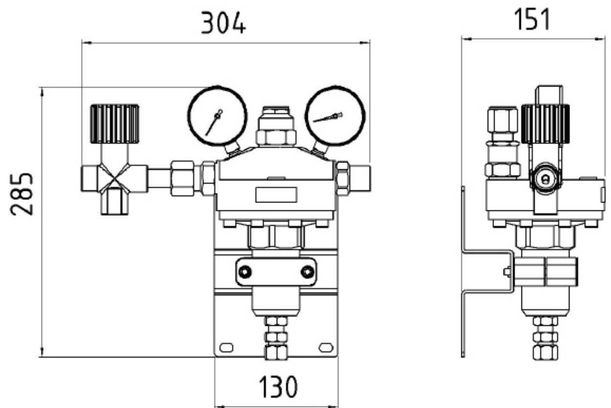
Ausführung 2 - einseitige Druckregelstation (links), auch in rechts lieferbar, Abmaße identisch.
