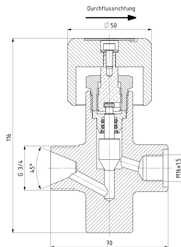
Ausführung 1: G 3/4" Kugel Konus X M16x1.5
