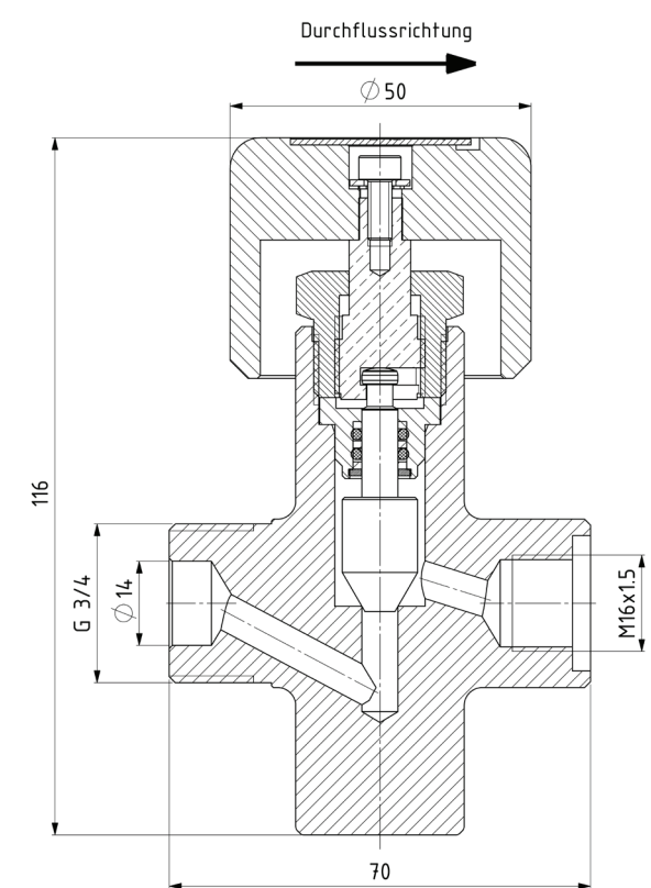
Ausführung 2: G 3/4" DIN 477 X M16x1.5
